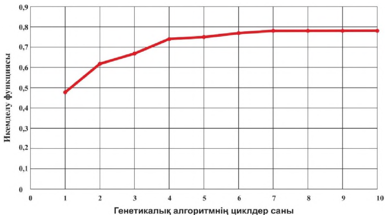
2.13-сурет. Өзірленген құрама генетикалық алгоритм үшін икемделу функциясының өзгерту кестесі
