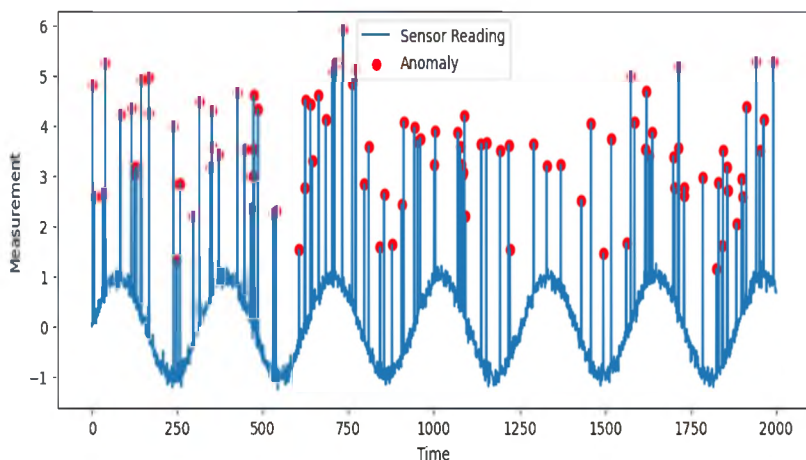
1.13-сурет. Аномалиялары бар синтетикалық IIoT сенсорлық деректері
