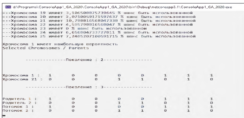
3.3-сурет. Генетикалық алгоритм көмегімен ақпараттық-коммуникациялық жүйе түйіні үшін ақпаратты қорғау құралдары іріктеуді онтайландыру процесін модельдеу нәтижелері бар терезе
