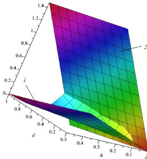
3.11-сурет. Екі беттің қиылысында құрылған мақсатты функцияны қалыптастыру: (1) – объектінің осалдығын сипаттайтын функция үшін және (2) - қорғау тарапынан ақпаратты қорғау құралдарына инвестициялаудың оңтайлы стратегиясын сипаттайтын функция.
