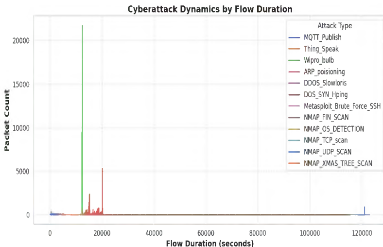
1.15-cyber. Flow Duration динамикасы
