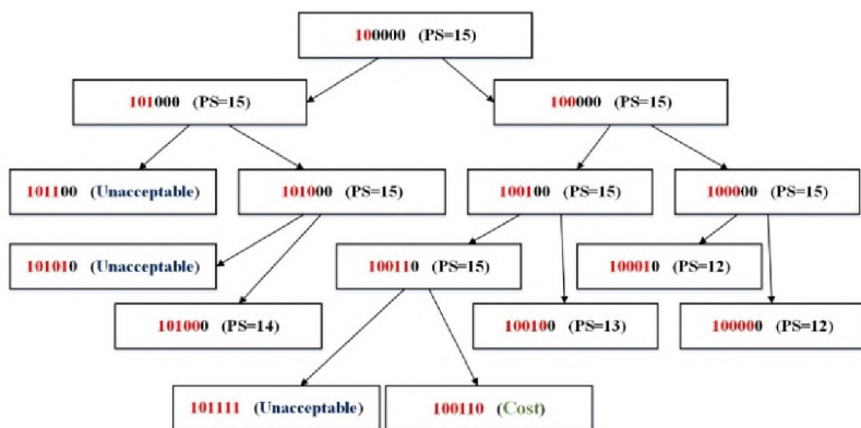
3.4-сурет. Генетикалық алгоритм мен ШБӨ-ны біріктірілген түрлендірілген алгоритм жұмысының иллюстрациясы
