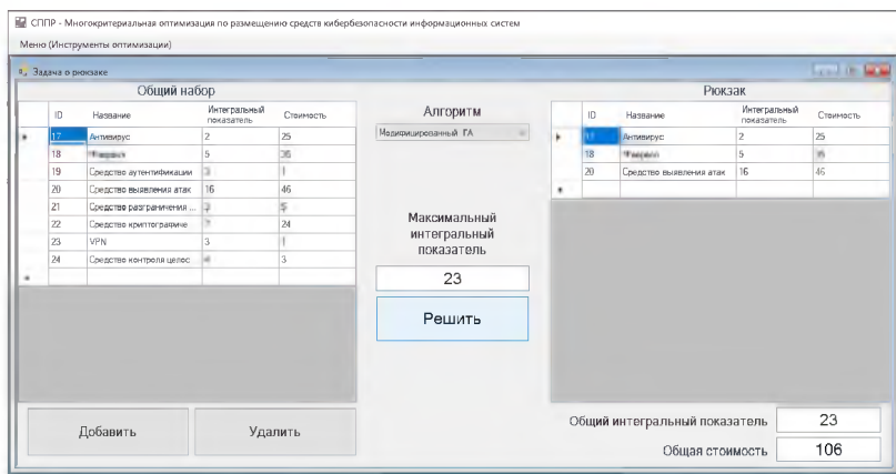
3.6-сурет. Шешім қабылдауды қолдау жүйесі модулі интерфейсінің жалпы түрі (модуль-түйін үшін ақпаратты қорғау құралдары құрамын тандау есебін шешу үшін генетикалық алгоритм қолдану)
